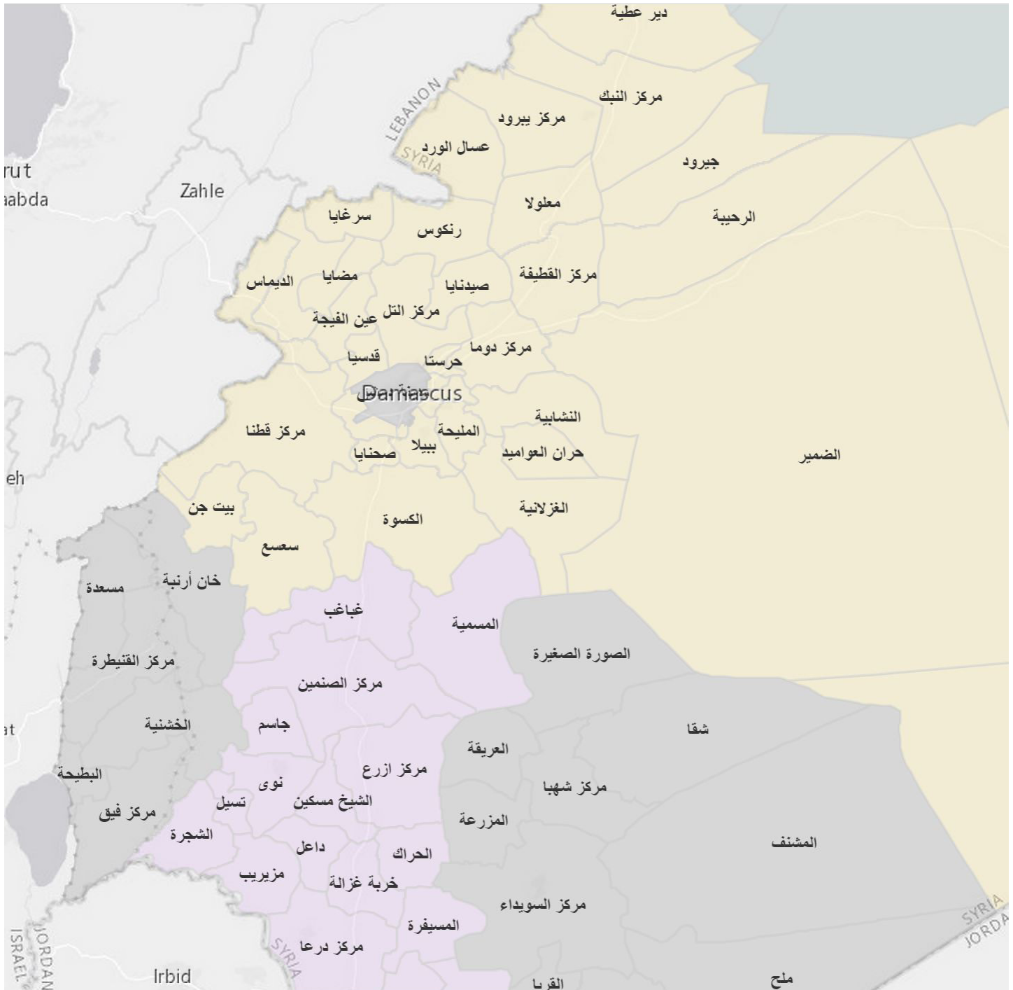
شكل ١٣: التقسيم الإداري لمناطق الجنوب السوري.
